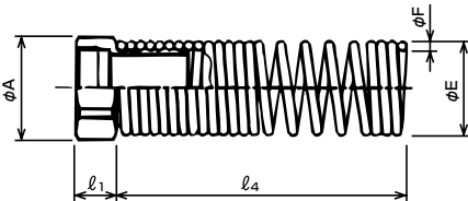
単位:mm
