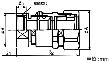
単位 : mm
