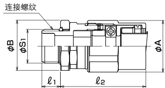
单位: mm
