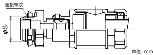
单位: mm
