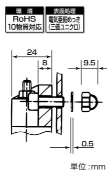
単位:mm
