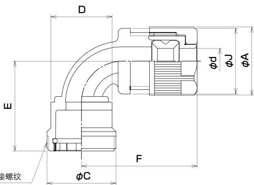
单位: mm
