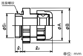
单位: mm
