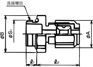
单位: mm
