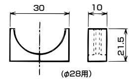
(φ28用)
