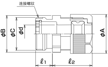
单位: mm
