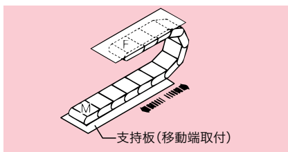
U:反動型
