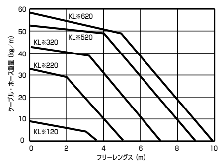
4.Type KL
