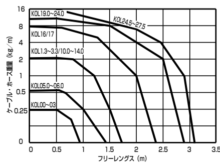
2.Type KOL
