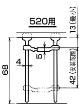
单位: mm
