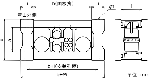
单位: mm
