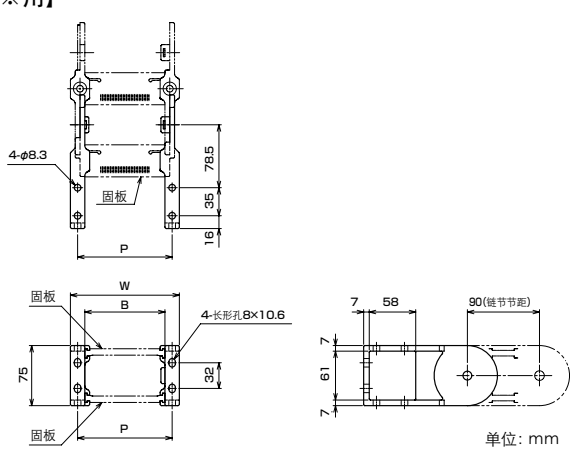
【PKK32※用】
