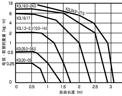
2.Type KOL
