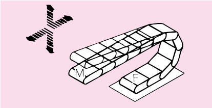
M: 多向型
