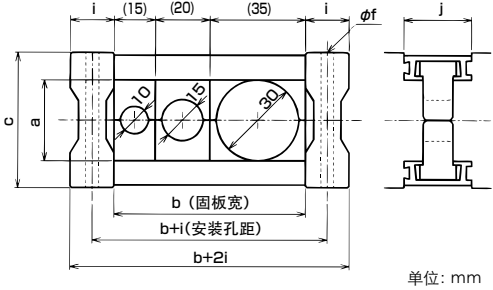
单位: mm
