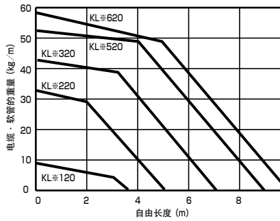
4.Type KL
