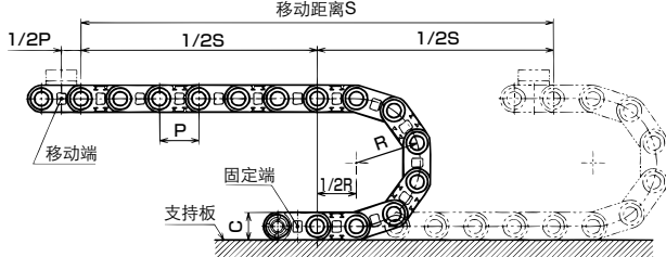
单位: mm
