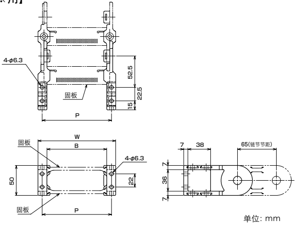
【PKK22※用】
