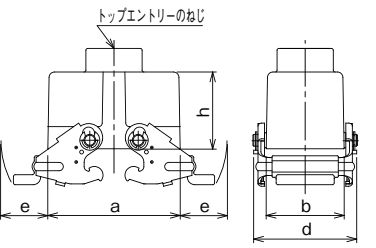
パッキンなし
