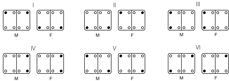
■ 2 インサート又は、2 モジュールフレームのガイドピン取付組合せ図
