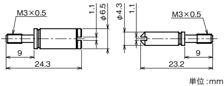
■ 1 インサート又は、1 モジュールフレームのガイドピン／ガイドブッシュ取付組合せ図
