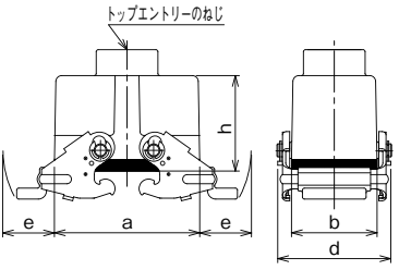
パッキン付き
