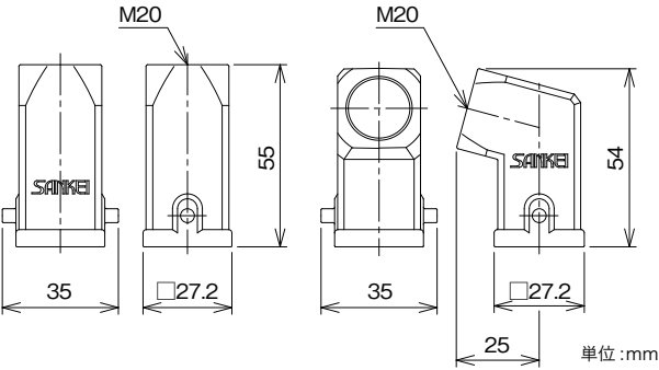
トップエントリー
