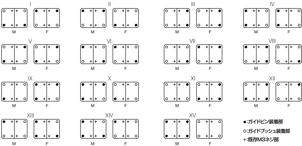
■ 2 インサート又は、2 モジュールフレームのガイドピン／ガイドブッシュ取付組合せ図
