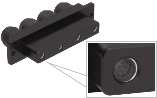
多極コネクタ製作 4芯一体型コネクタ
