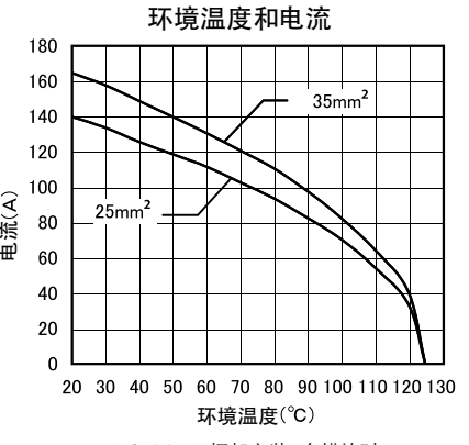
YSF※24B框架安装3个模块时
