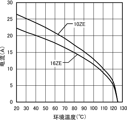
电线尺寸2.5mm 2
