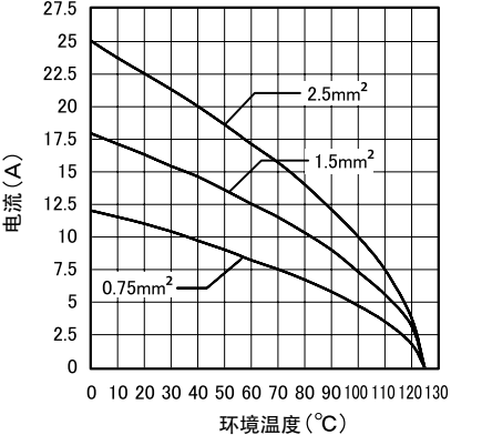
环境温度和电流
