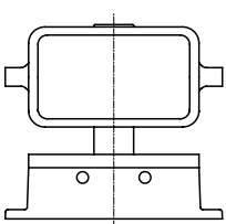
有销底座
