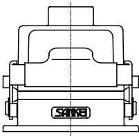
底座 (箱型)
