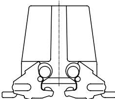
中转外罩 (外罩用)
