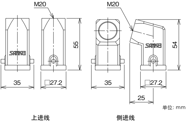
上进线
