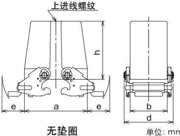
无垫圈
