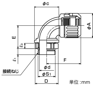
単位:mm
